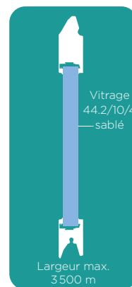
Double vitrage
