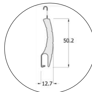
Coupe de la lame
