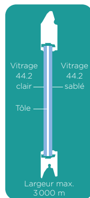
Vitrage + tôle
