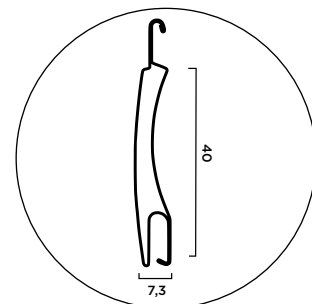
Coupe de la lame
